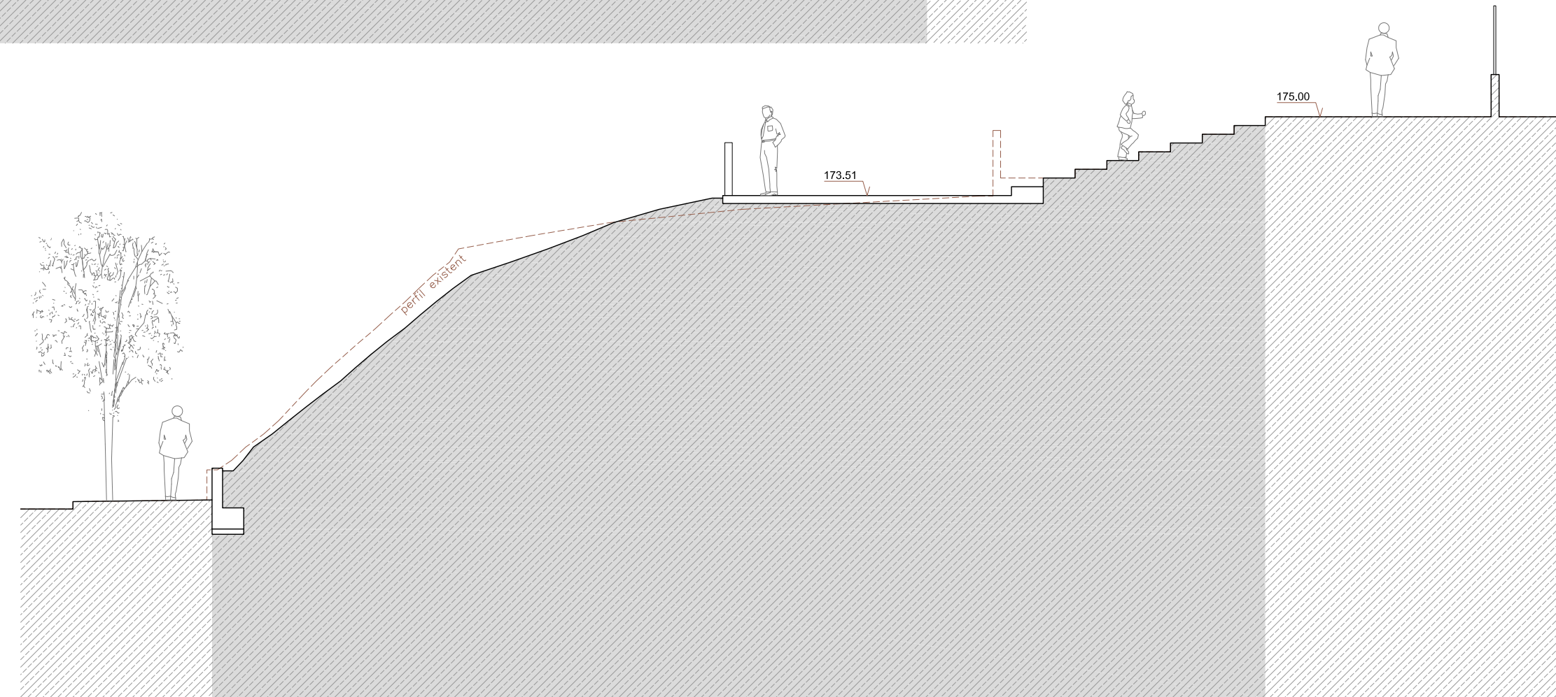
SECCIÓ S1
