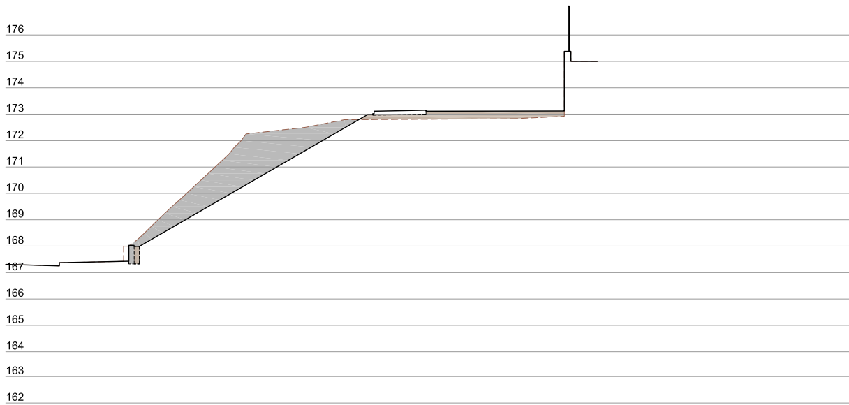
Perfil P-2 (4)
