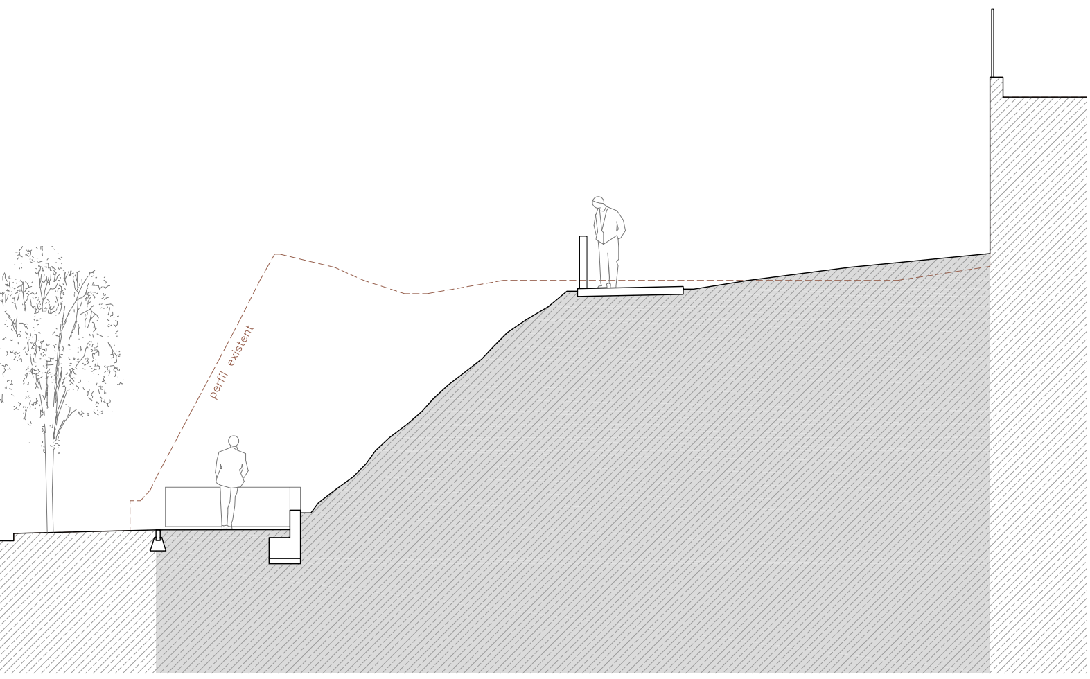
SECCIÓ S2
