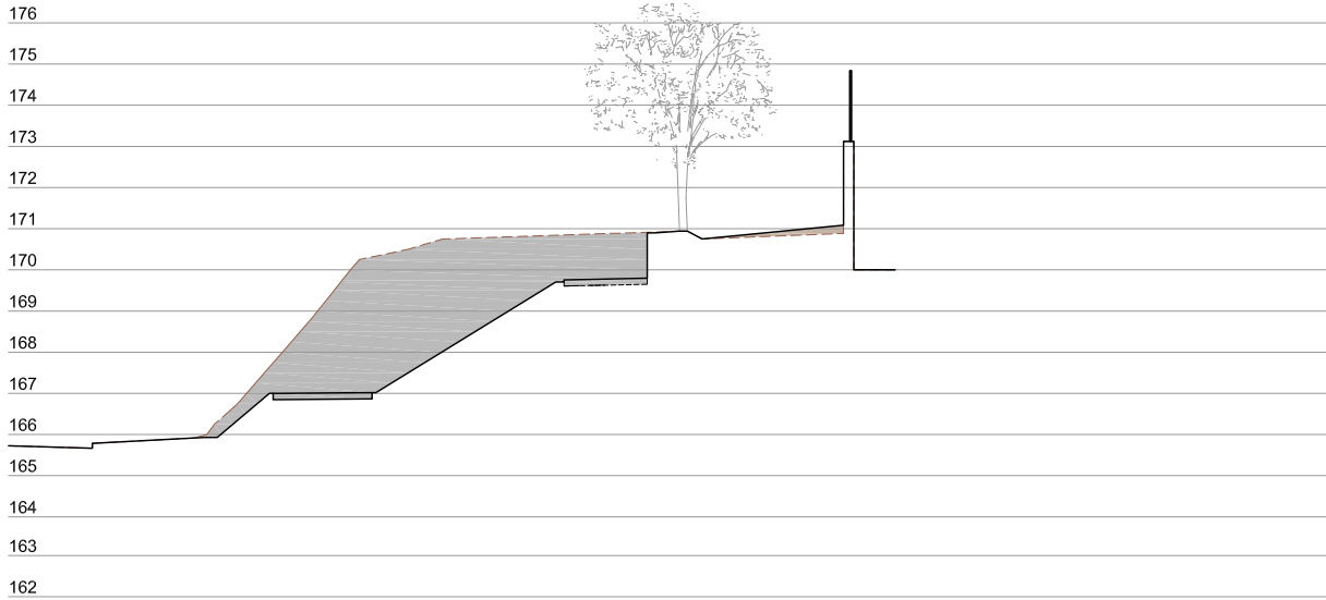
Perfil P-7 (2)
