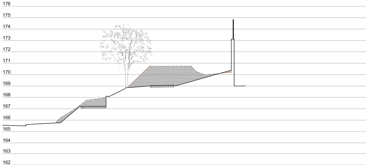
Perfil P-9 (2)
