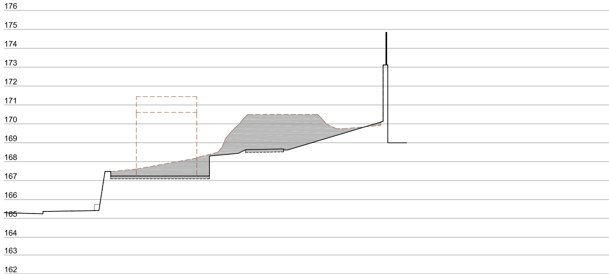
Perfil P-10 (3)
