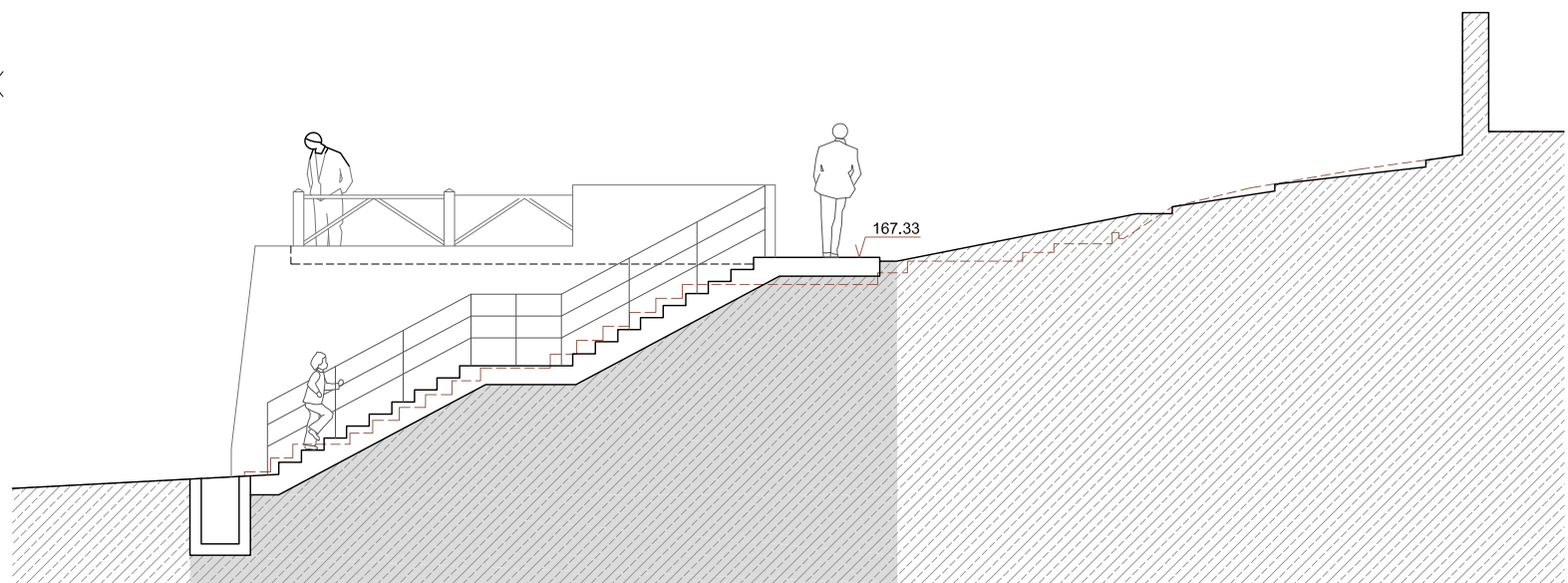
SECCIÓ S6
