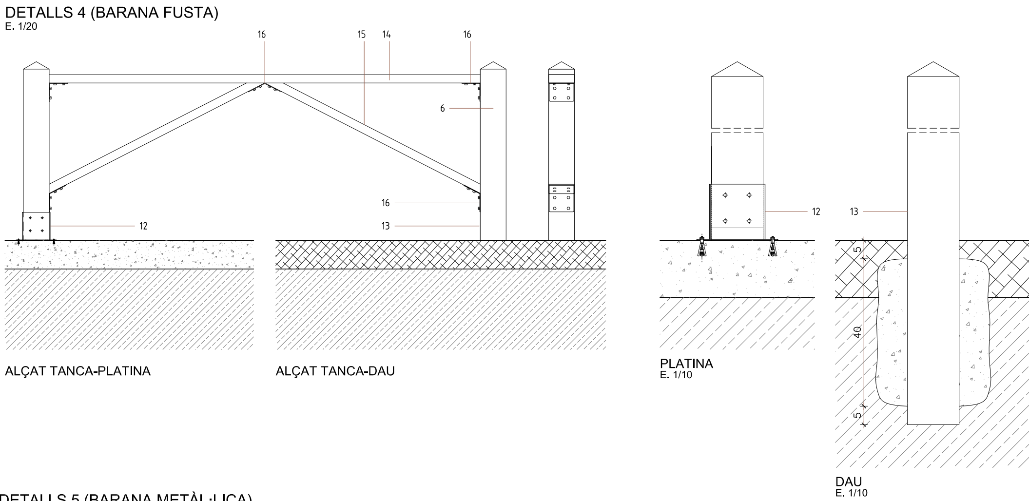
DETALLS 5 (BARANA METÀL·LICA)
