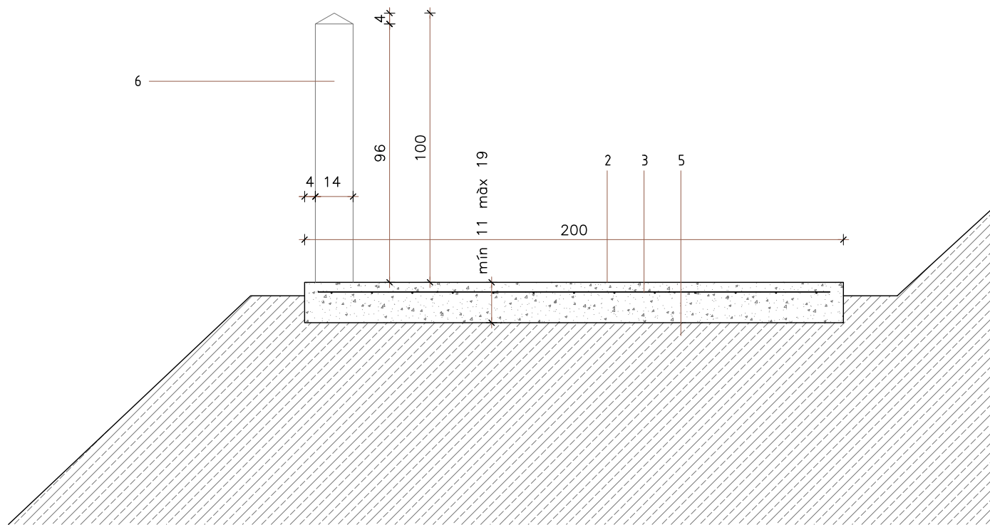
SECCIÓ TRANSVERSAL (D2.2)
