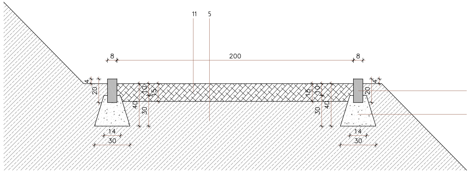
SECCIÓ TRANSVERSAL (D1.2)
