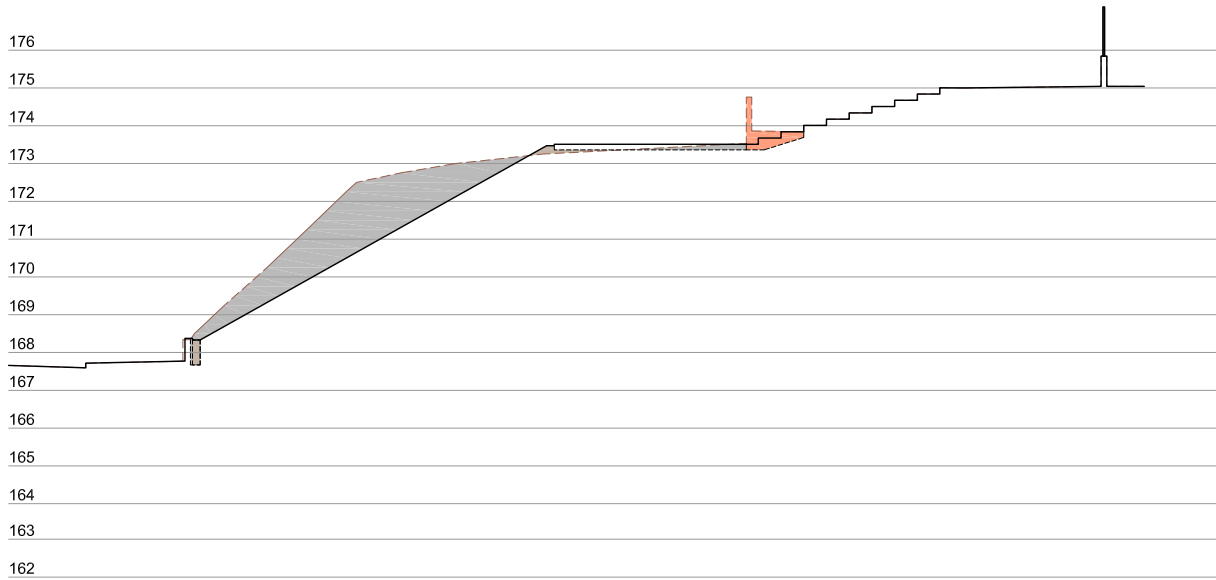
Perfil P-1 (2)
