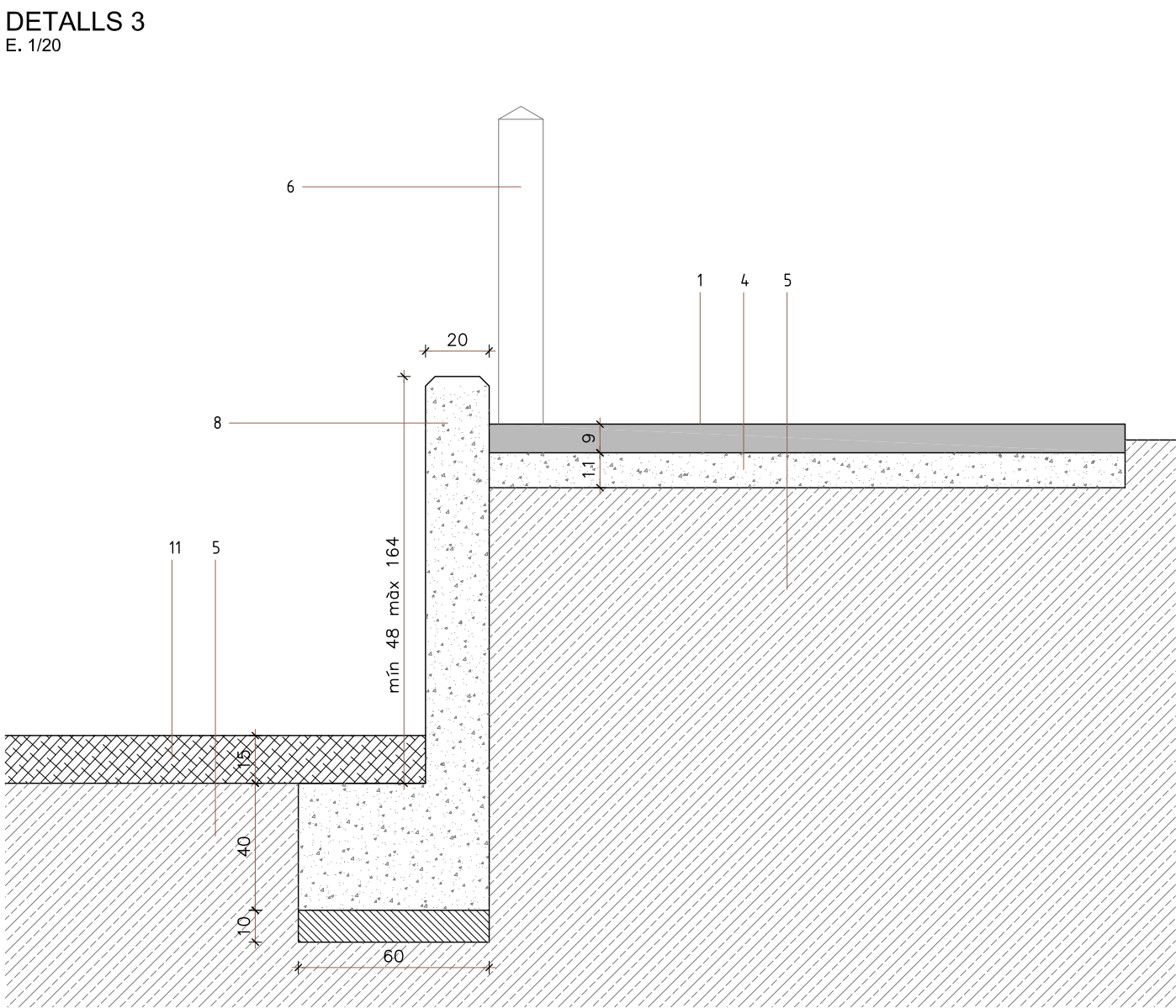
SECCIÓ TRANSVERSAL (D3.1)
