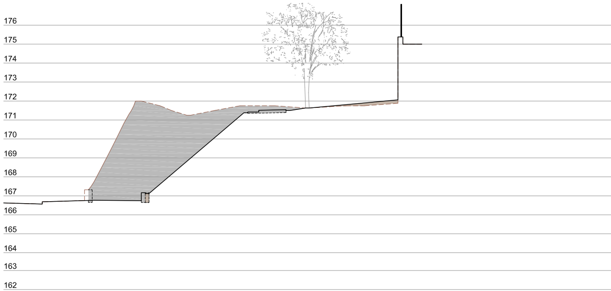
Perfil P-4 (4)
