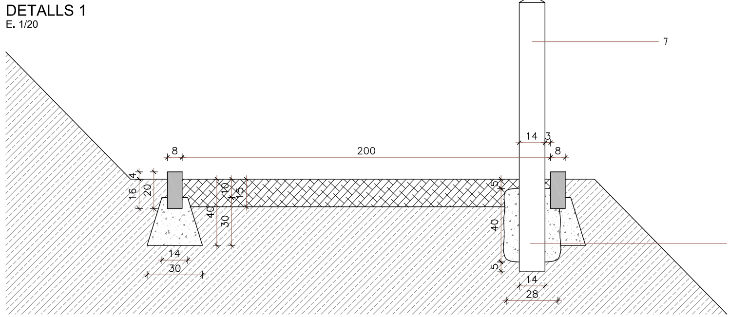
SECCIÓ TRANSVERSAL (D1.1)
