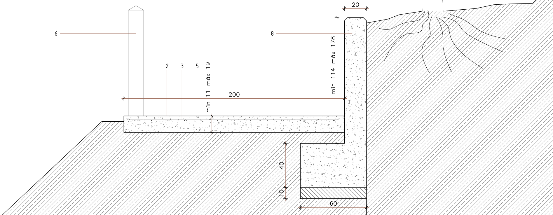
SECCIÓ TRANSVERSAL AMB CONTENCIÓ (D2.3)
