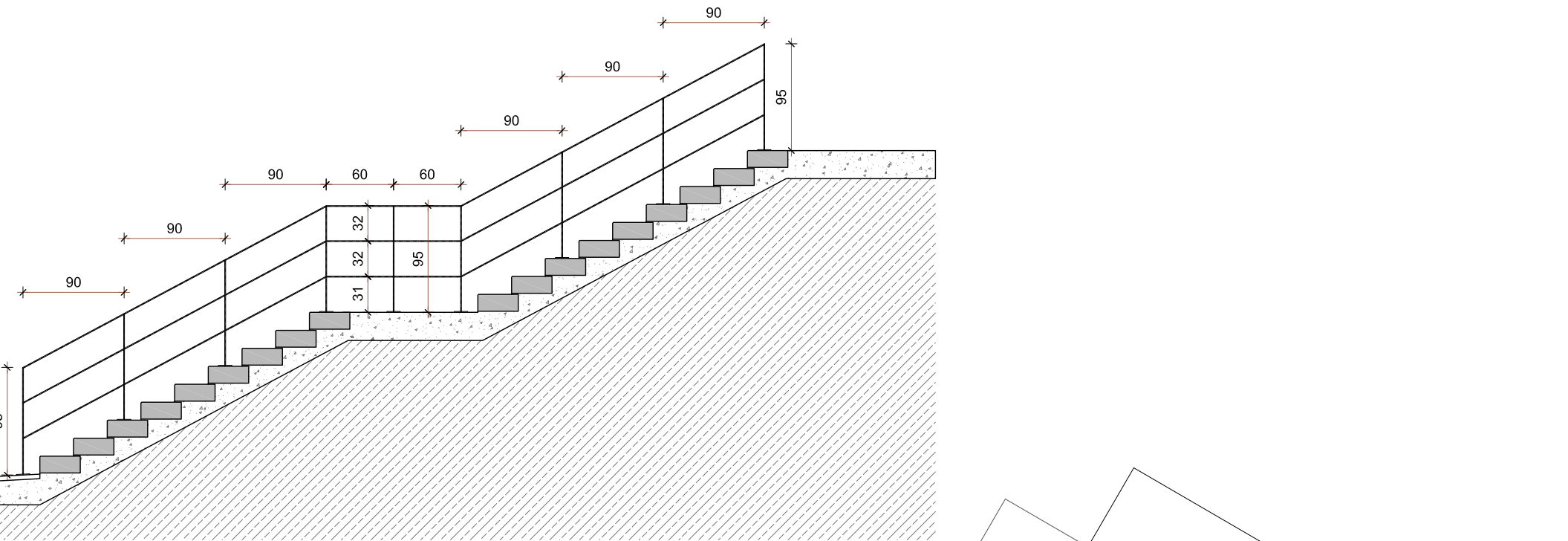
SECCIÓ 1
