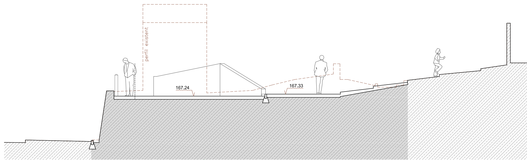
SECCIÓ S7
