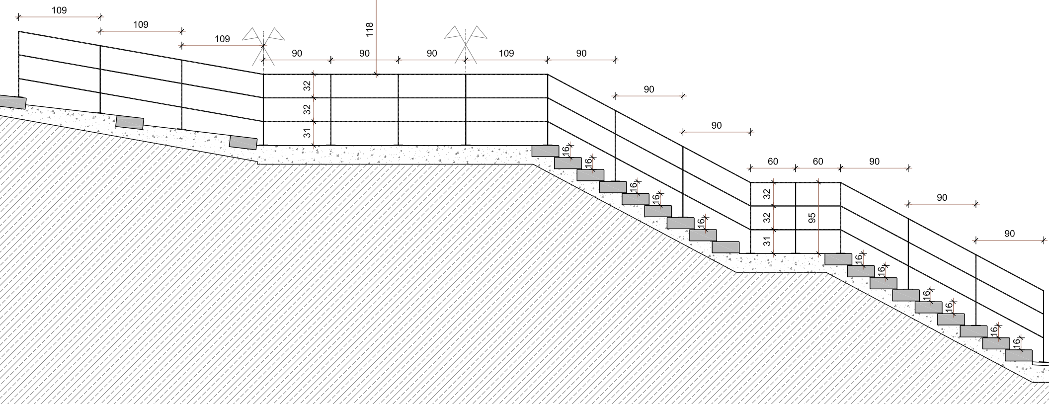
SECCIÓ 2
