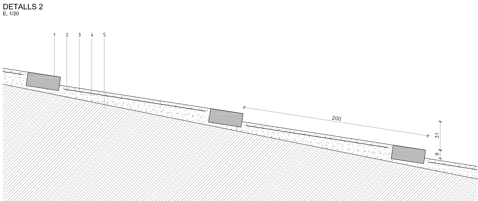
SECCIÓ LONGITUDINAL (D2.1)
