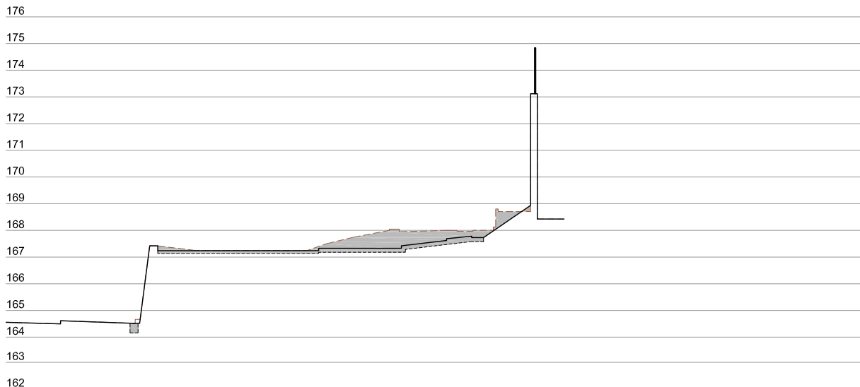
Perfil P-12 (3)
